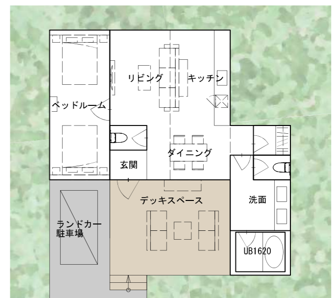
スタンダード (59㎡) 1:100 20ftコンテナ×4
